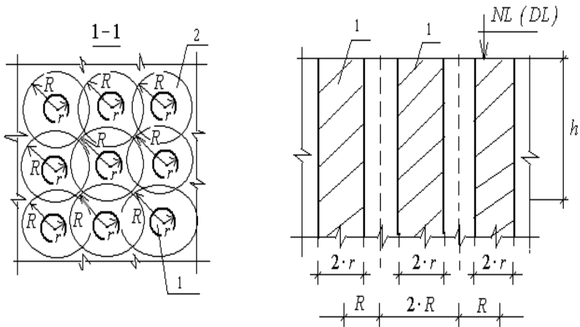
Рис. 1 – Расположение скважин коллекторов тепловых насосов в плане (схема). 1 – скважина коллектора; 2 – зона влияния коллектора; r – радиус скважины коллектора; R – радиус зоны влияния коллектора; h – глубина, на которой определяется температурное поле и изменение тепловой энергии.
