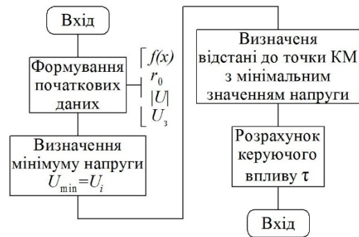
Рис. 6. Алгоритм роботи системи керування
