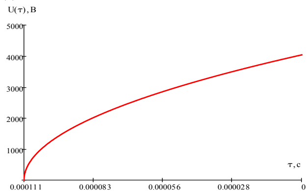
Рис. 2. Вихідна характеристика підсилюючого пункту
