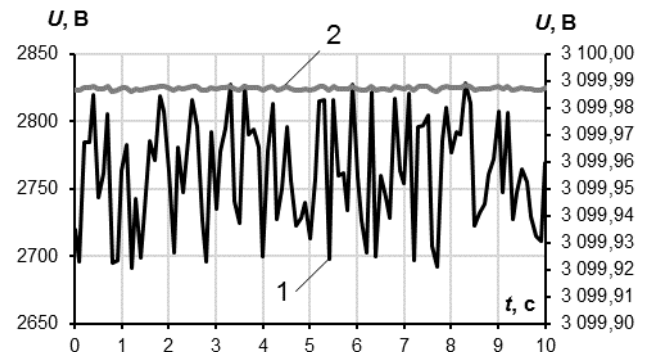
Рис. 8. Графік зміни напруги на струмоприймачі електровоза: 1 – до підключення підсилюючого пункту; 2 – після підключення підсилюючого пункту
