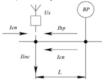
Рис. 5. Ділянка контактної мережі з підсилюючим пунктом
