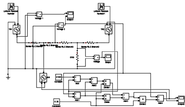
Рис. 7. Імітаційна модель системи керування
