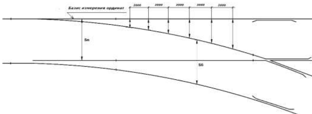
Рис. 2. - Методика ординатного контроля
