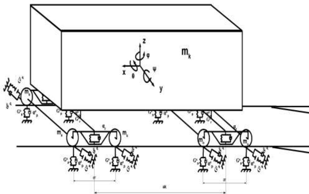
Рис. 7. Схема пространственной математической модели грузового полувагона
