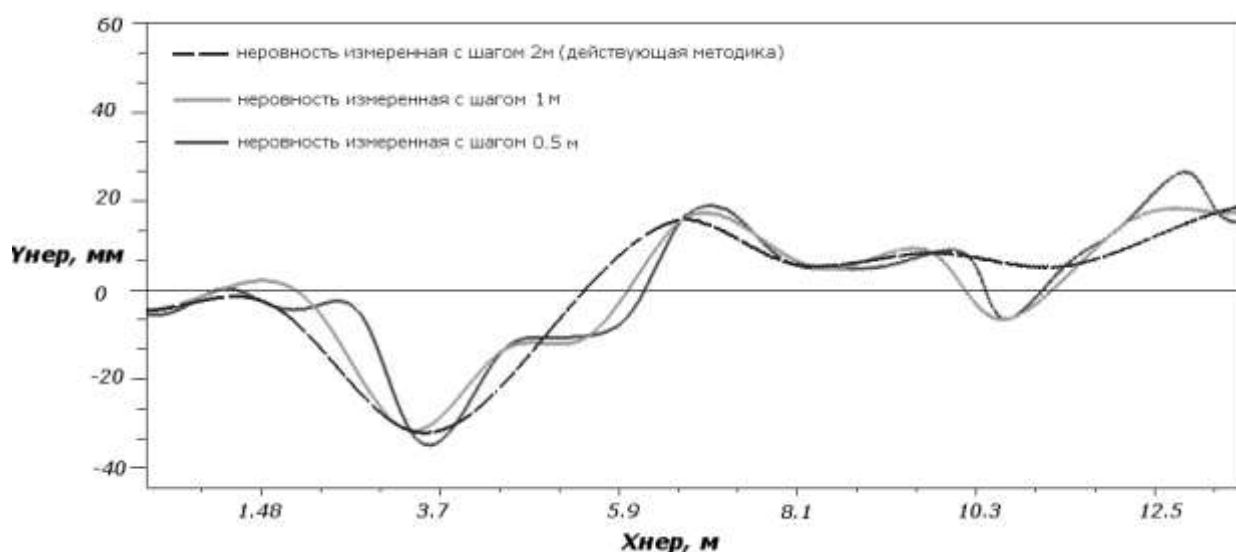
Рис. 6. Горизонтальные неровности в пределах упорной нити
