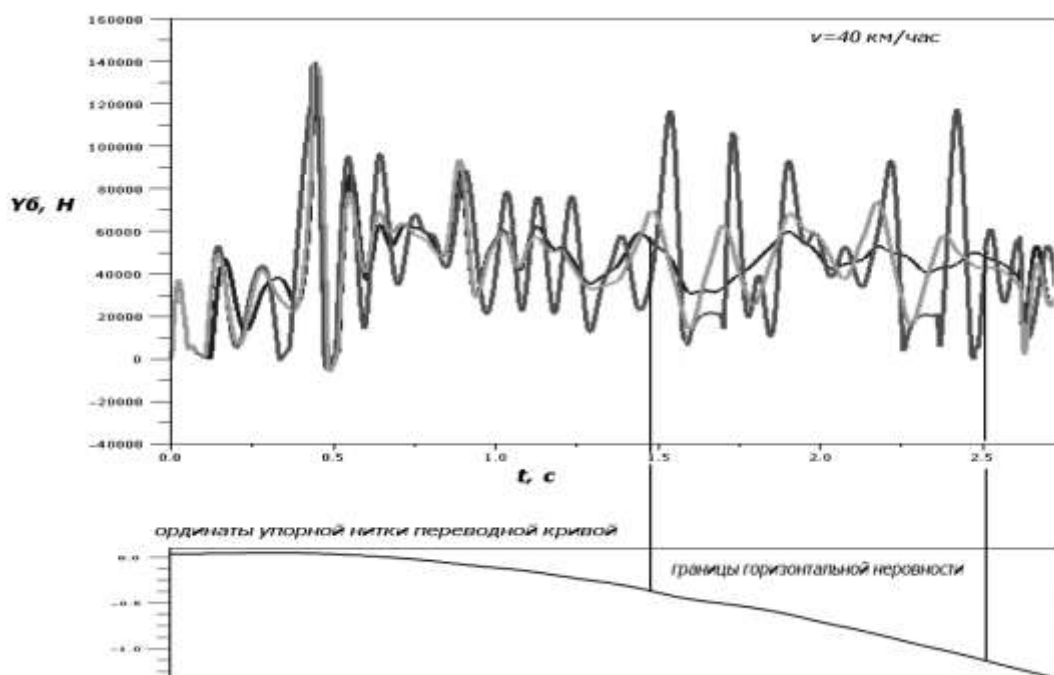
Рис. 8. Результаты моделирования при различном шаге промера ординат
