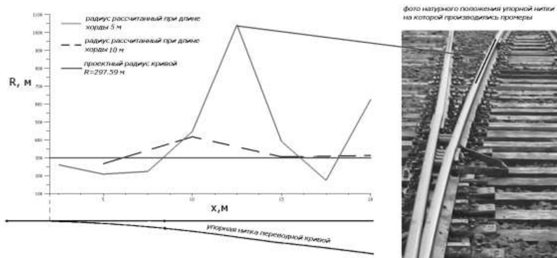
Рис. 1. Натурный радиус переходной кривой при различной длине хорды.
