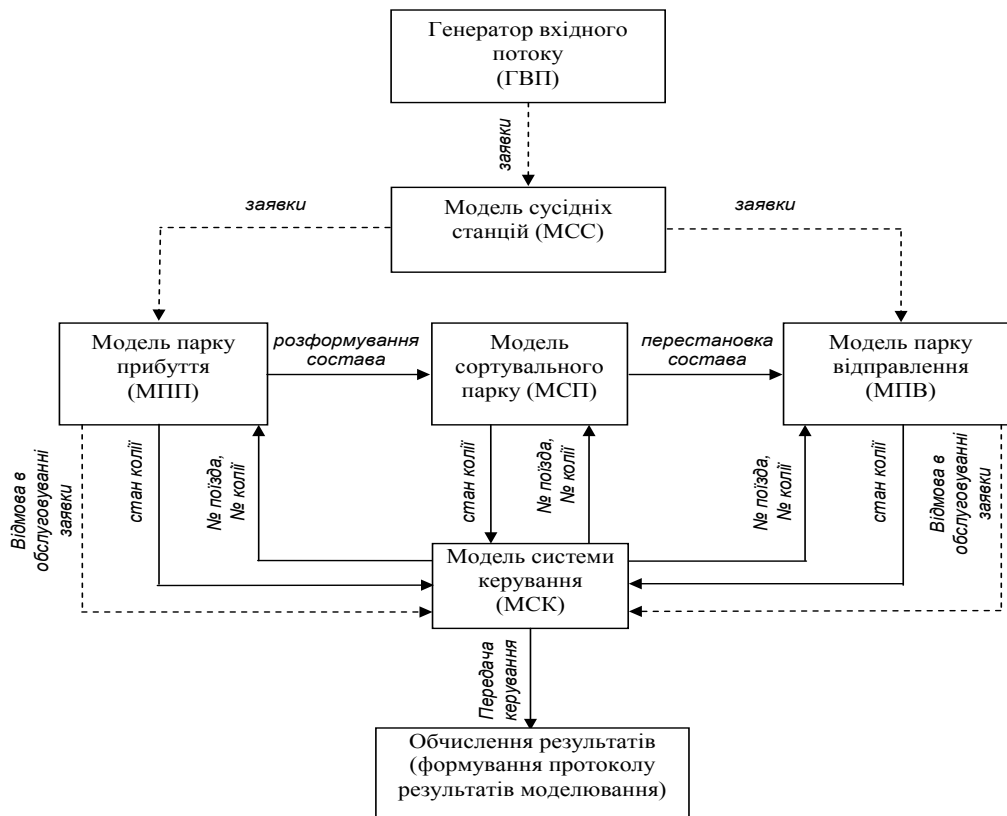
Рис. 1. Загальна структура функціональної моделі станції
