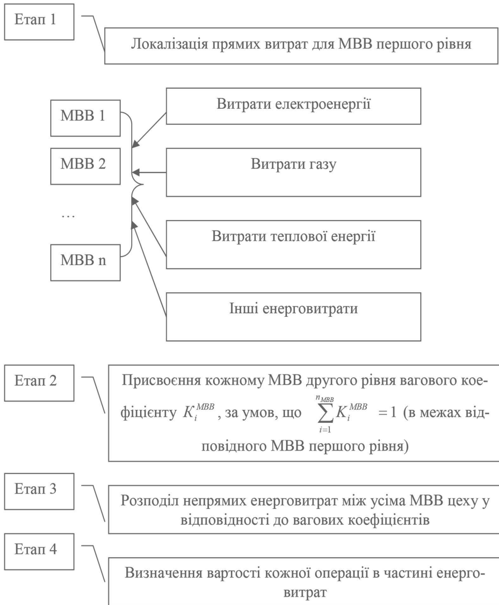
Рис. 2. Послідовність локалізації і поопераційного розподілу енерговитрат трубного підприємства
