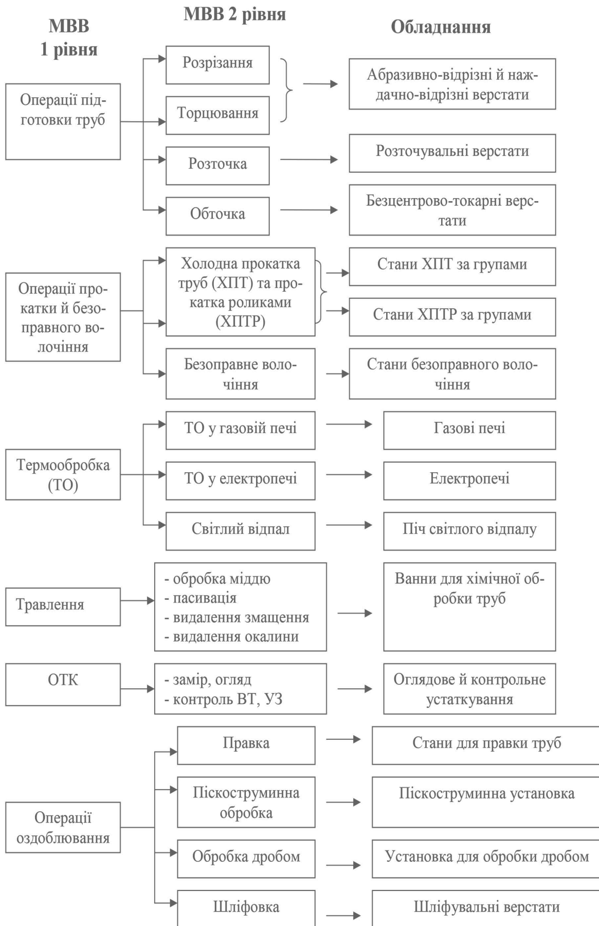
Рис. 1. Операційні центри цеху основного виробництва трубного підприємства за групами обладнання
