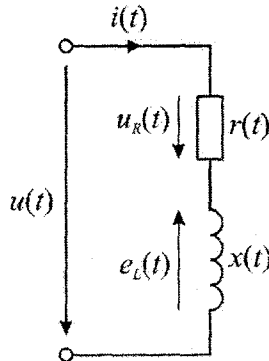
Рис. 1. Схема заміщення активно-індуктивного навантаження
