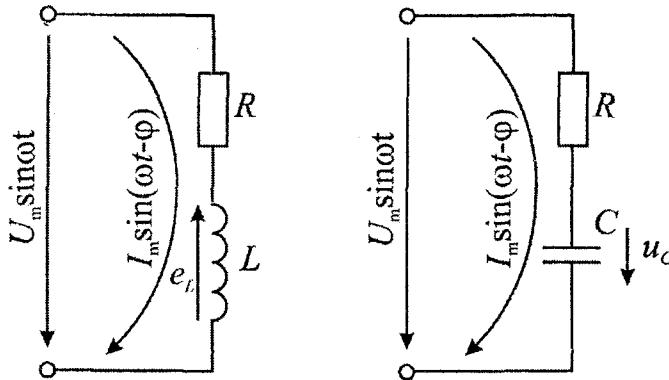
Рис. 5. Схеми заміщення активно-індуктивного та активно-ємнісного навантаження
