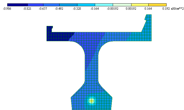
Рис. 6. Изополя нормальных напряжений в сечениях блока пролетного строения расположенных за анкером
