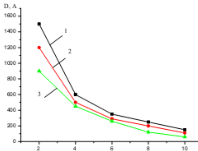
Рис. 2 Залежність розмірів блоків мозаїки від значення \beta при катодних густинах струму 1 – 20 А/дм 2 ; 2 – 30 А/дм 2 ; 3 – 40 А/дм 2
