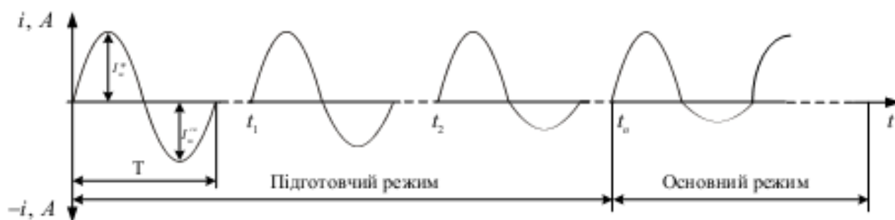
Рис. 1 Часова діаграма асиметричного струму
