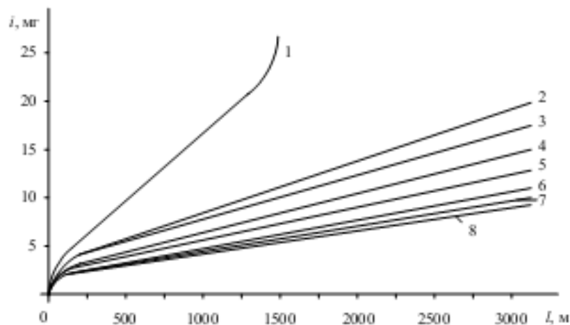
Рис. 5 Залежність зносу електроосадженого заліза при сухому терті від пробігу при питомому тиску 2 МПа. Контролю – сталь 45 загартована с.ч. 1 – Сталь 45 загартована с.ч.; 2-8 – шарувате покриття
