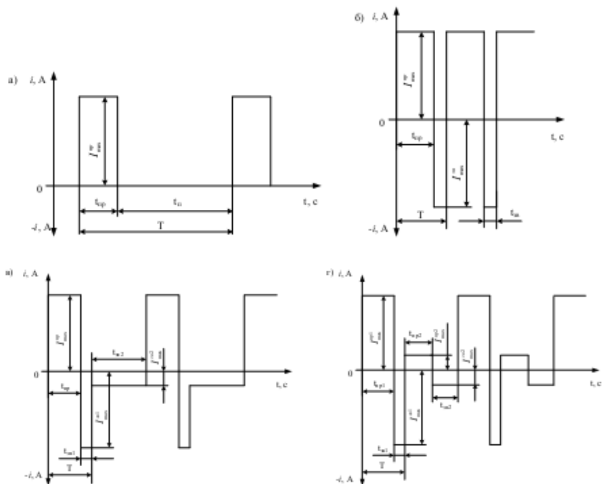
Рис. 3 Часові діаграми струмів а) імпульсного уніполарного; б) імпульсного реверсивного; в), г) імпульсного із поєднаннями (термін автора)
